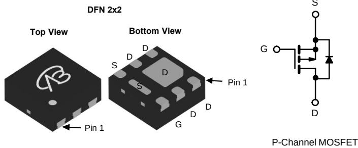
P-Channel MOSFET
