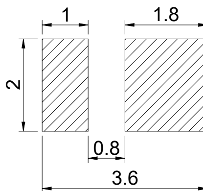
焊盘建议图
