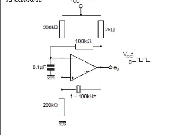
方波振荡器
