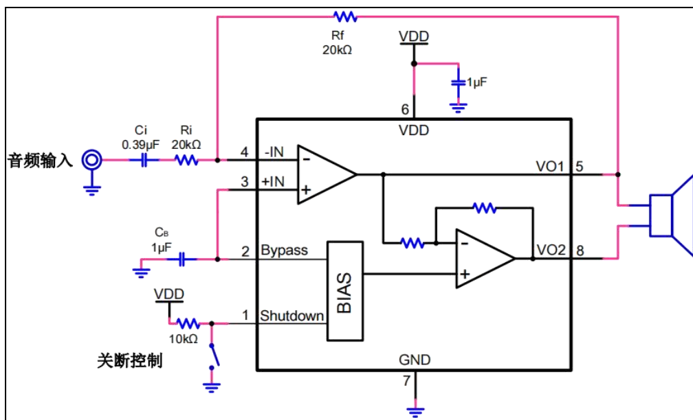
图 2. TPA6204 单端输入模式电路图
