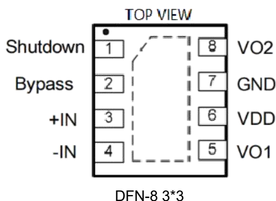
图 1. TPA6204 的管脚定义图
