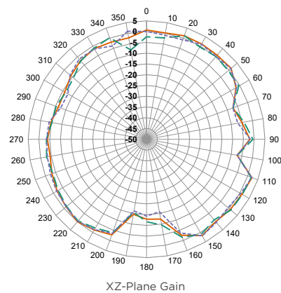
XZ-Plane Gain
