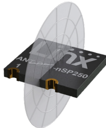
YZ-Plane Gain
