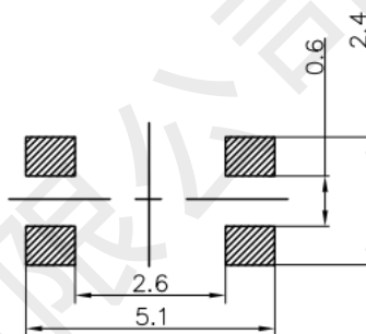
安装参考尺寸
