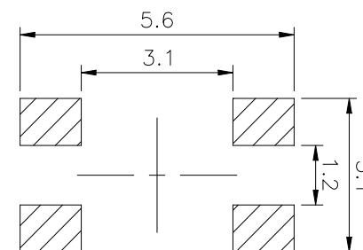
PCB. 焊接图
