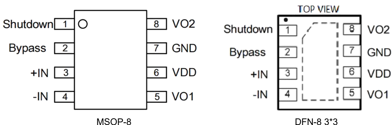
图 1. TPA6203 的管脚定义图
