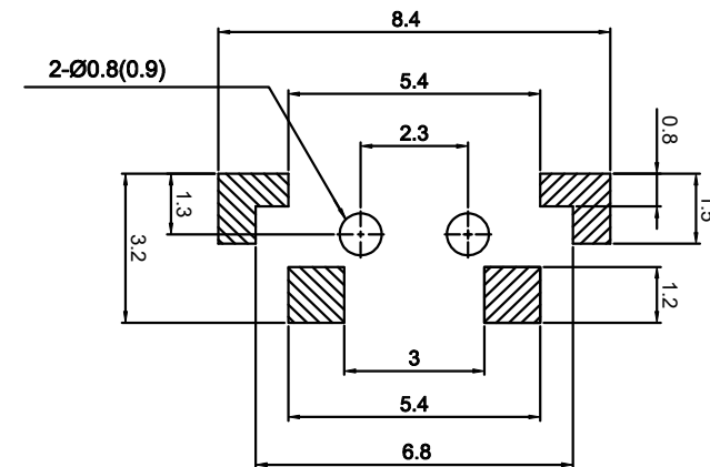
PCB. 焊接图
