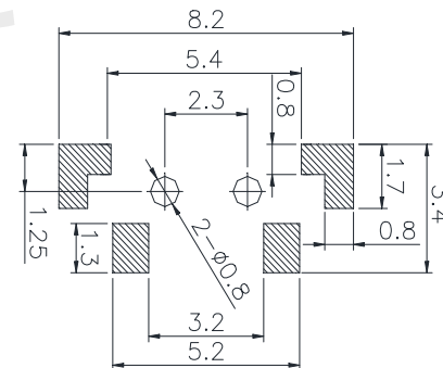
PCB. 焊接图
