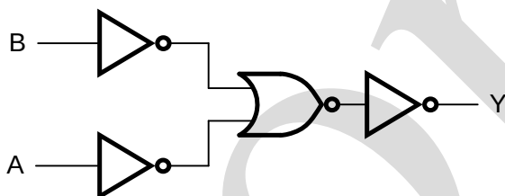
图 3 逻辑框图
