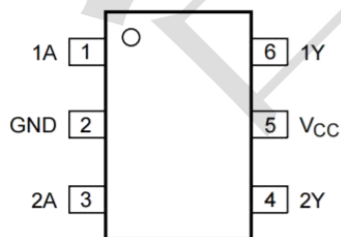
SOT363
