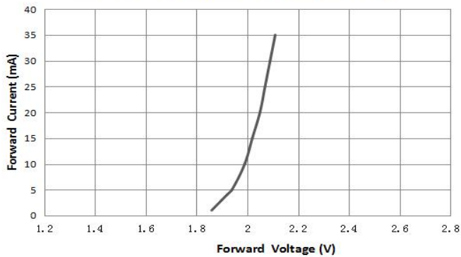
伏安特性曲线
