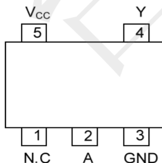
SOT353
