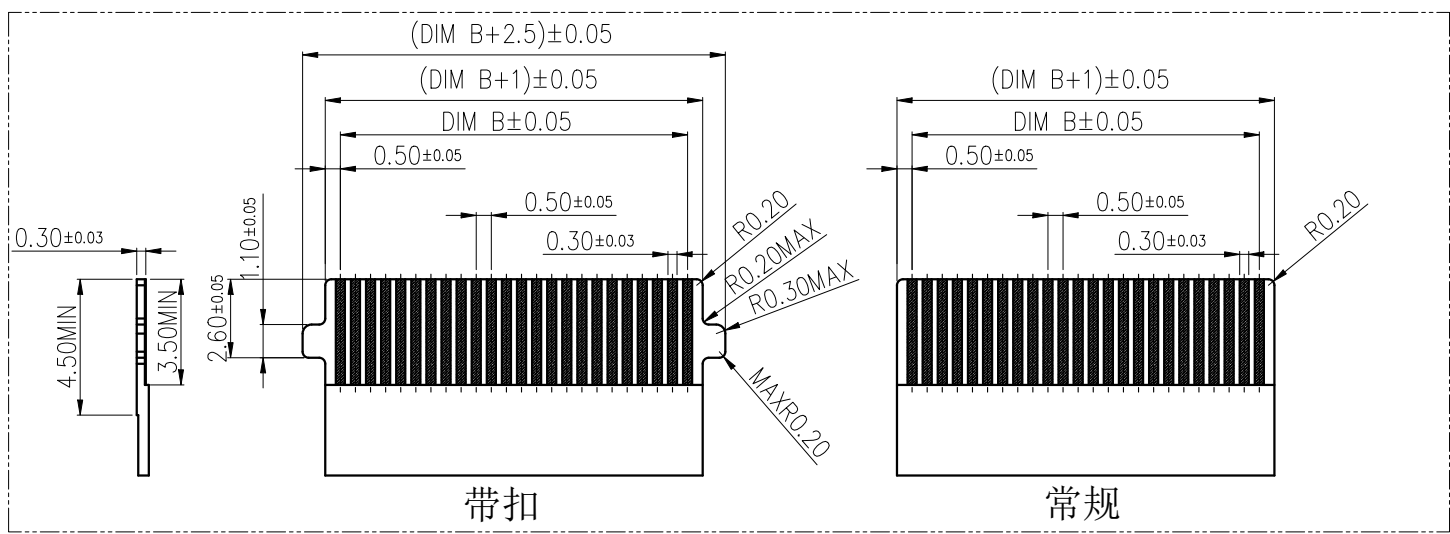
适用线路板 (PCB LAYOUT)
