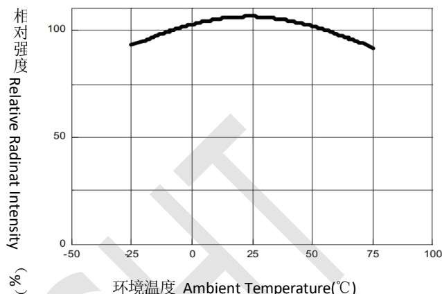
输出特性
