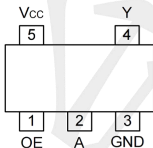
SOT23-5
