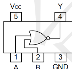
SOT23-5/ SOT353
