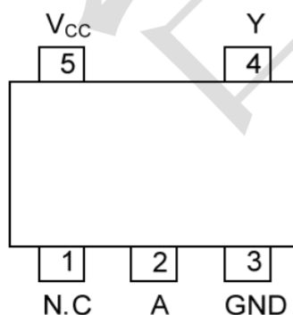
SOT23-5
