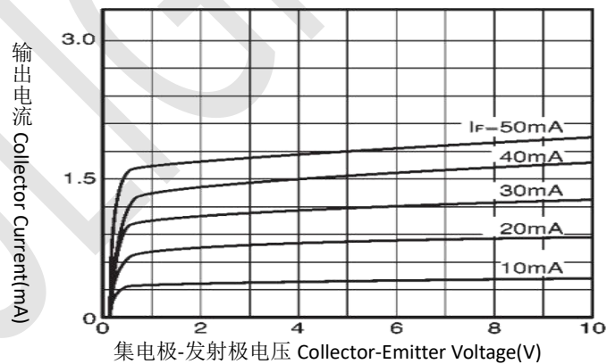
输出特性 Output Characteristics
