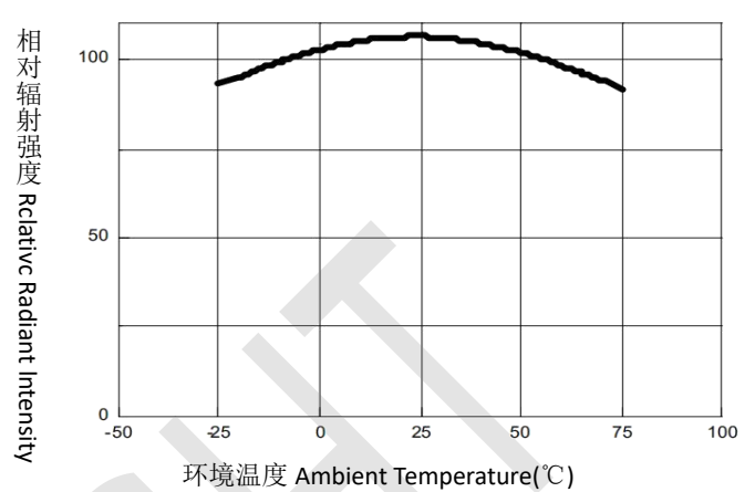
输出特性 Output Characteristics
