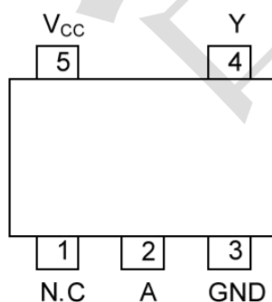
SOT23-5
