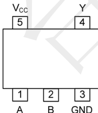
SOT353
