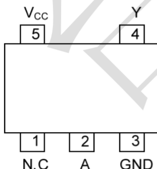
SOT353
