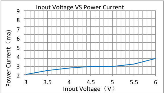
图4 : Input Voltage VS. Power Crrnt
