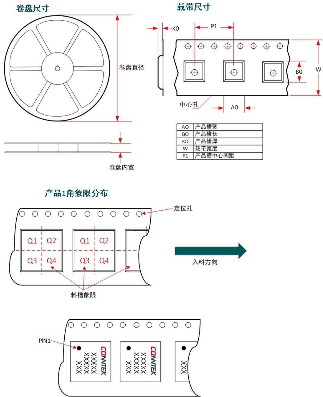
图 16: QFN-16L 卷盘载带尺寸
