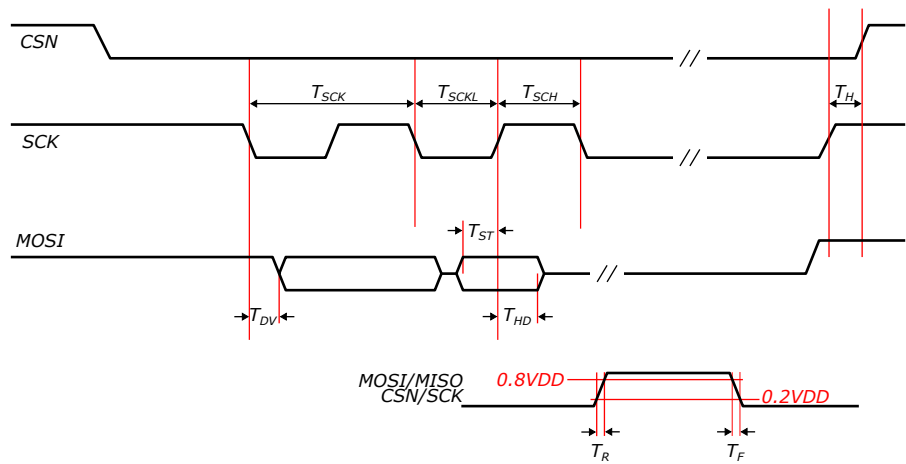
图 7: SPI 时序图
