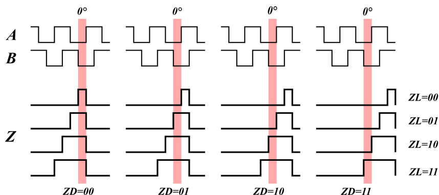
图 10: ABZ 的 Z 信号的宽度 ZL 和位置 ZD
