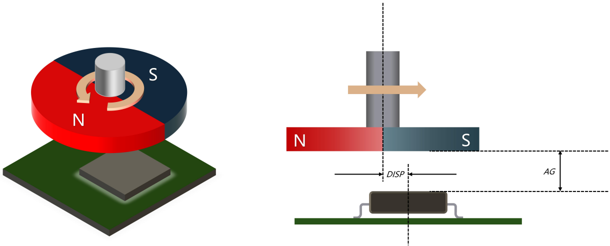
图 4: 在轴磁铁芯片摆放位置
