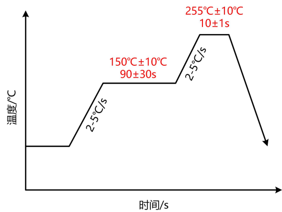
图 19: 焊接温度曲线
