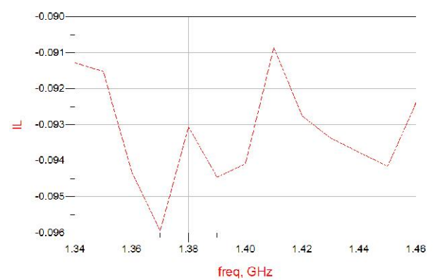
Figure 10. MHC1400M30 IL
