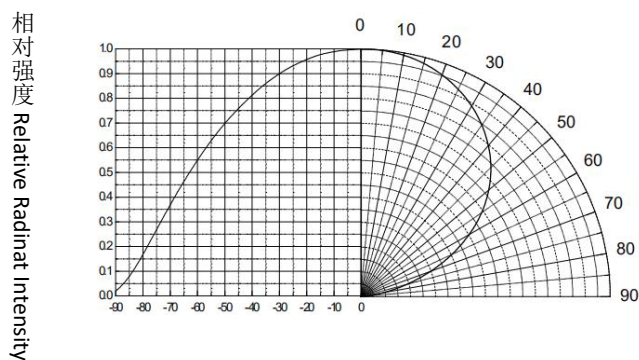
相对辐射强度与角位移的关系 Relative Radiant Intensity vs. Angular Displacement
