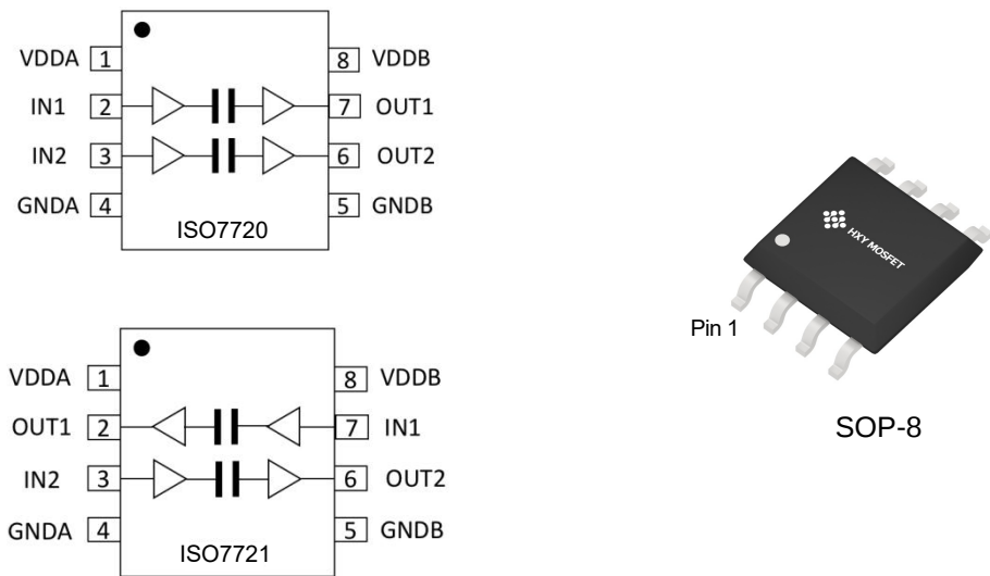
图 2-1 ISO772xSOP-8 封装顶部视图
