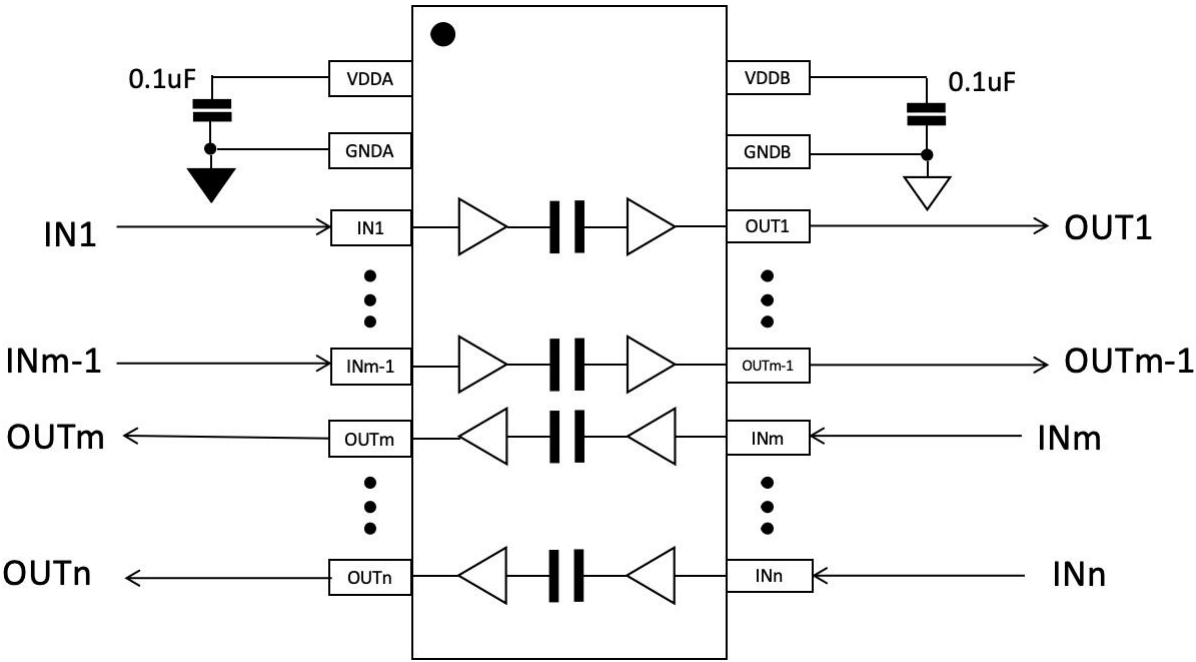
图 6-1 SOW-16 ISO772x典型应用电路
