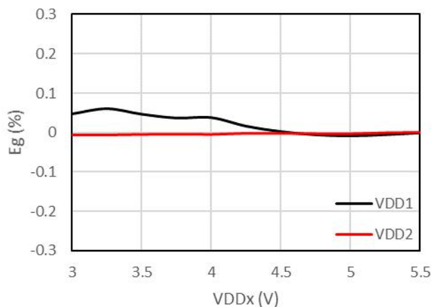
图 3-26 增益误差 vs 供电电压 (AMC1301)
