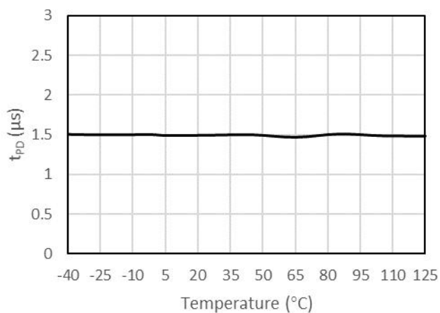
图 3-19 输入输出信号延时 vs 温度
