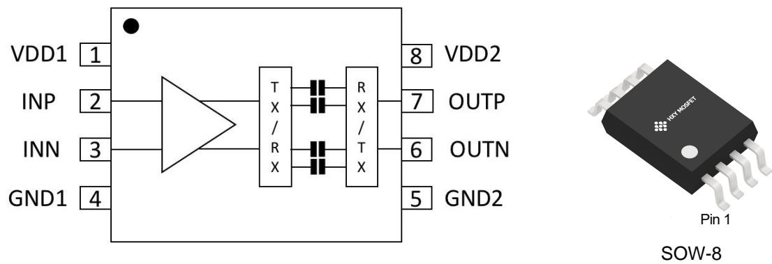
图 2-1 AMC130x引脚配置表
