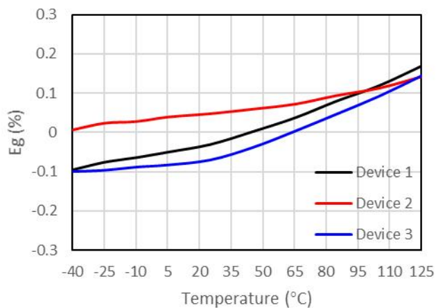
图 3-25 增益误差 vs 温度 (AMC1301)
