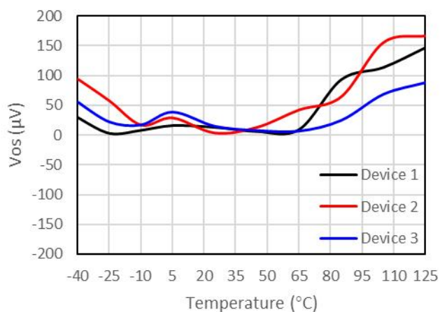
图 3-27 输入失调电压 vs 温度 (AMC1301)
