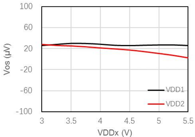
图 3-4 输入失调电压 vs 供电电压 (AMC1300)
