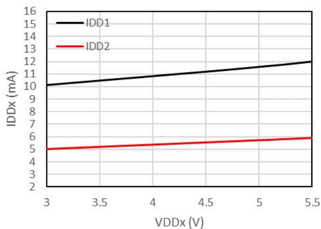
图 3-30 供电电流 vs 供电电压 (AMC1301)
