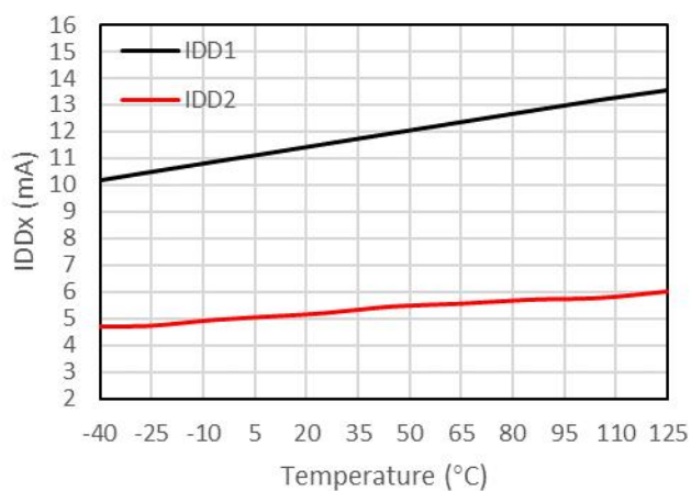
图 3-29 供电电流 vs 温度 (AMC1301)
