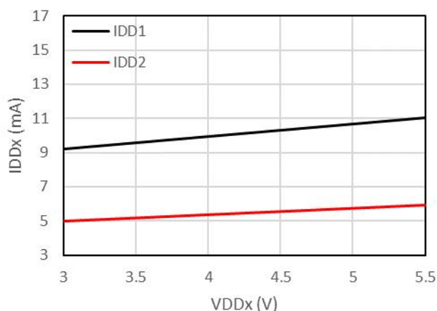
图 3-22 供电电流 vs 供电电压 (AMC1300)
