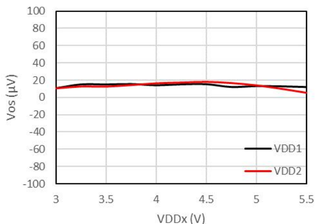
图 3-28 输入失调电压 vs 供电电压 (AMC1301)
