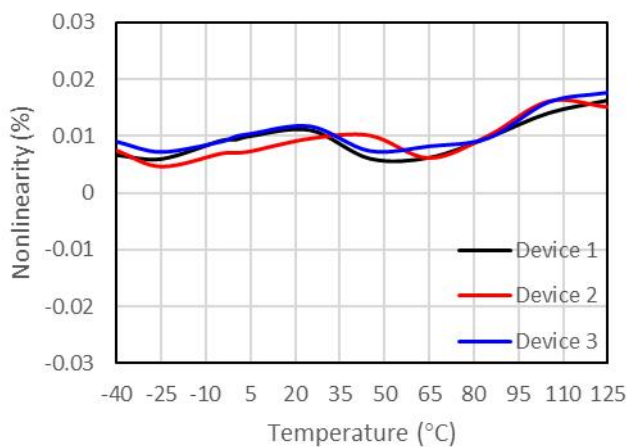
图 3-23 非线性度 vs 温度
