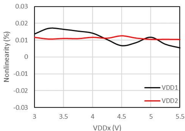
图 3-24 非线性度 vs 供电电压
