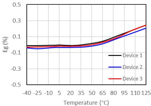
图 3-1 增益误差 vs 温度 (AMC1300)
