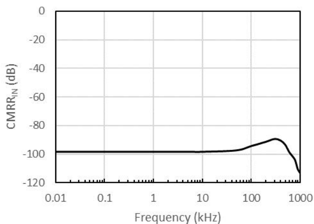
图 3-11 输入共模抑制比 vs 频率
