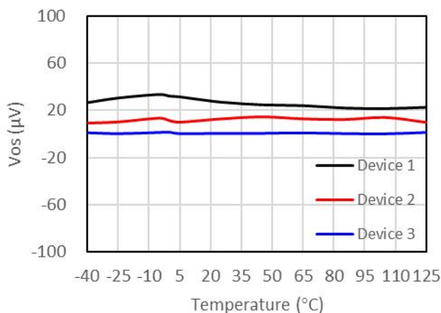
图 3-3 输入失调电压 vs 温度 (AMC1300)
