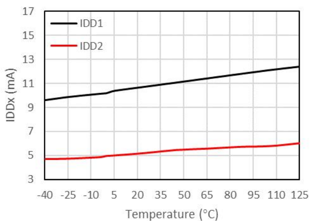
图 3-21 供电电流 vs 温度 (AMC1300)
