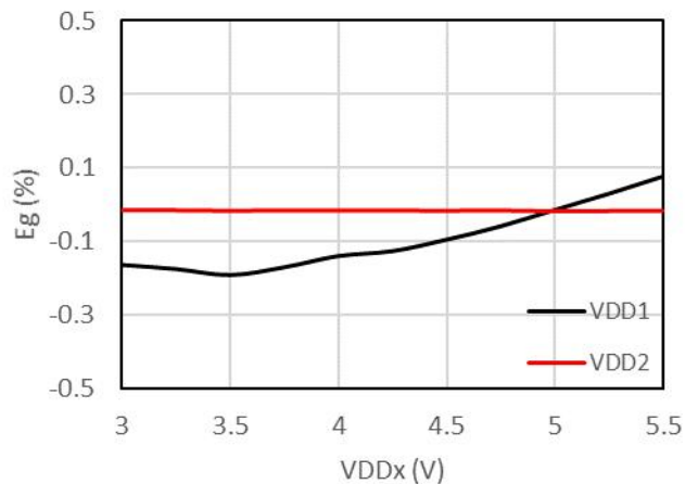
图 3-2 增益误差 vs 供电电压 (AMC1300)
