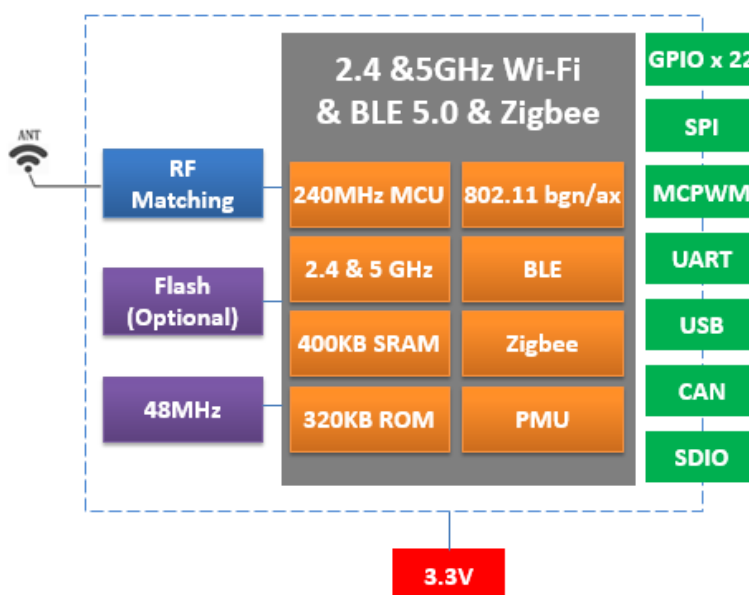
Fig.1.1 ESPC5-32E Module Structure
