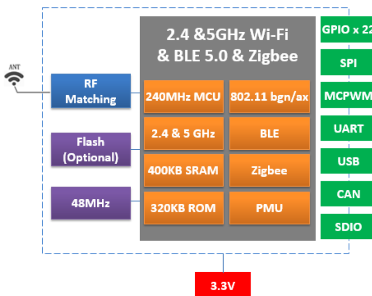
Fig.1.1 ESPC5-32 Module Structure
