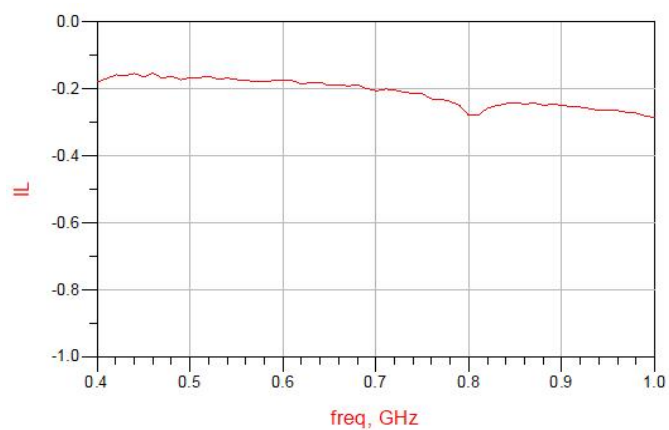
Figure 10. MHC0410L03 IL
