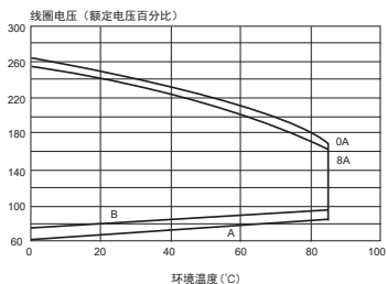
线圈工作范围曲线
