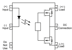
DIP-6
