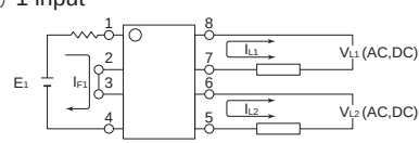
(2) 1 input
