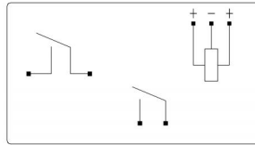
KT206-N MA 双线圈 Humbucker
