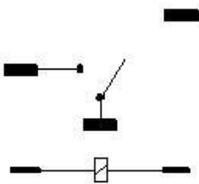
M：常开型 Form A
