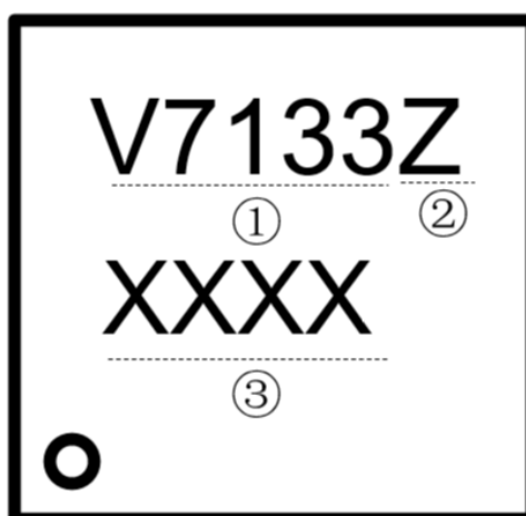
SOT23-6标识示意图
