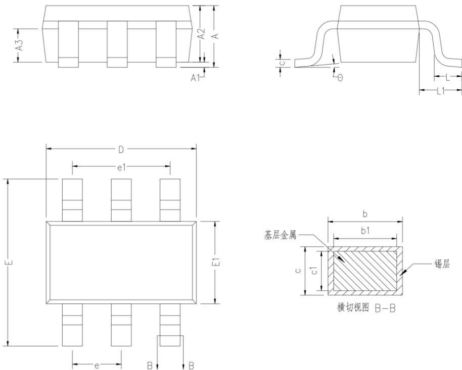
SOT23-6
