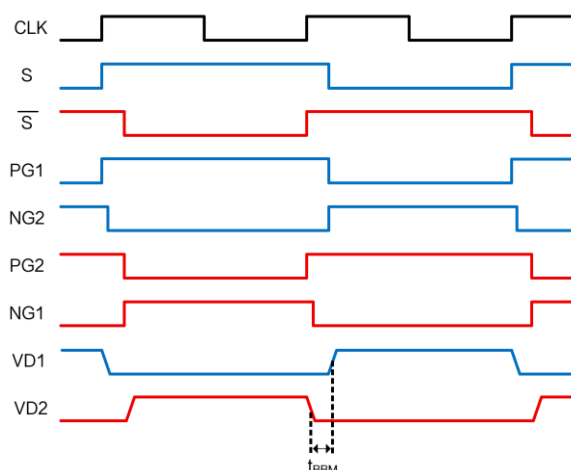
图 1. 驱动时序图
