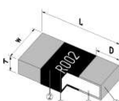
四位数白色标记 Four digit white marking (2512 < R004 大电极 large electrode)
