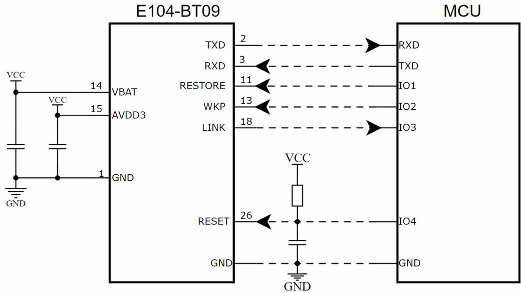
图 4-1 推荐电路
