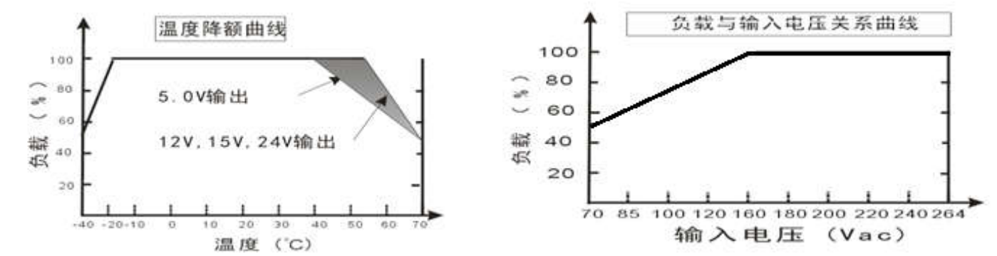
降额曲线图
