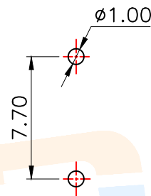
PCB Layout(Pattern Side)
