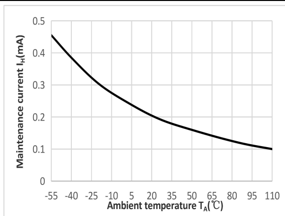
图 9 抑制状态泄漏电流 vs 环境温度
