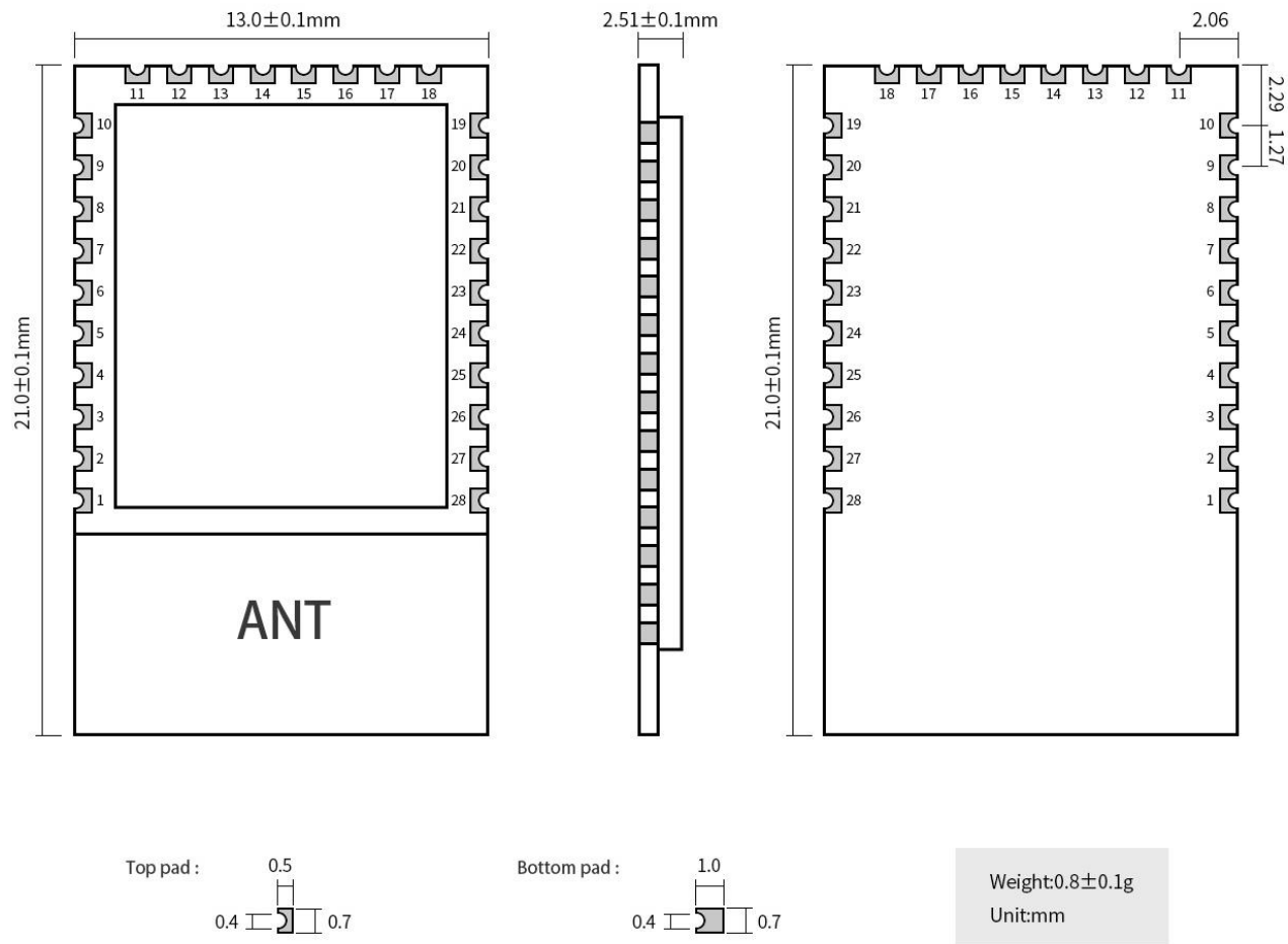
图 1 E104-BT40 引脚尺寸图
