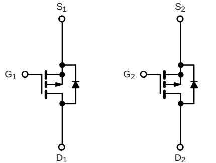
P-Channel MOSFET
