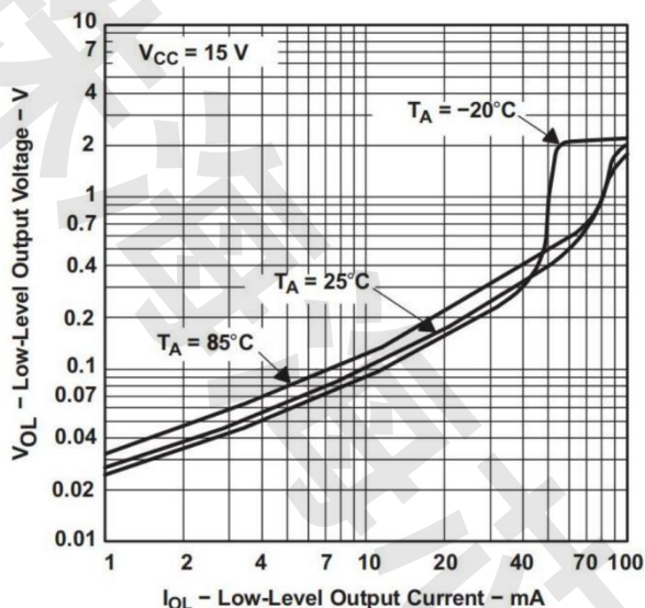
V_{CC}=15\text{V} ，低电平输出电压 VS 低电平输出电流
