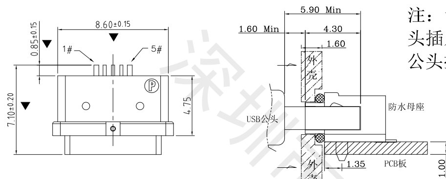
组装示意图
