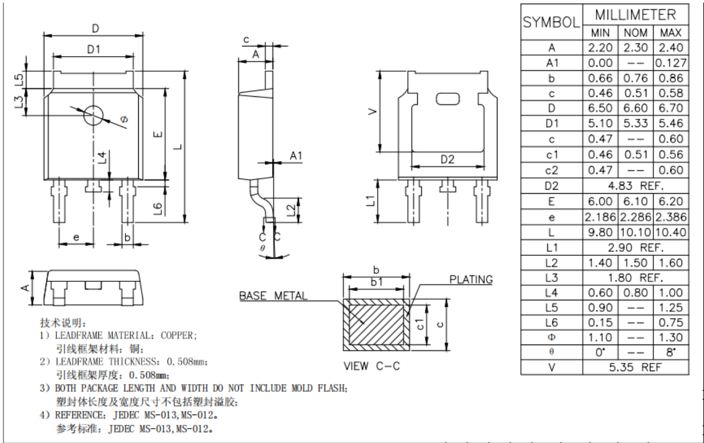
Figure4. TO-263
