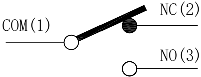
电路图
