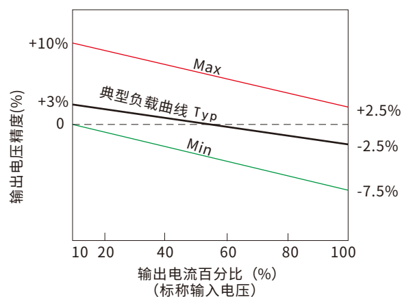
误差包络曲线图 5Vdc输出
